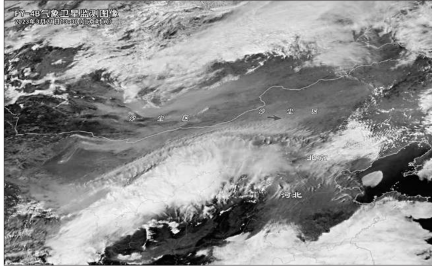
风云四号气象卫星监测今年以来强度最强沙尘过程的图像。 中国气象局供图
