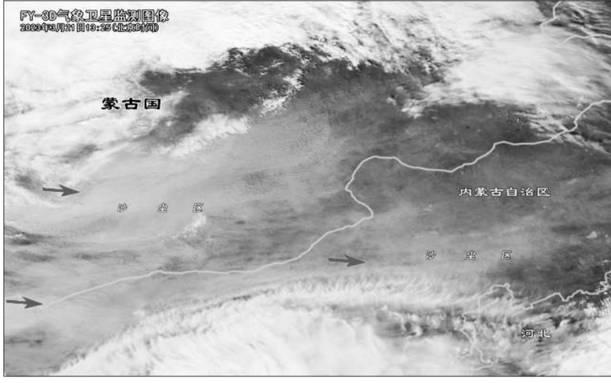
风云三号气象卫星监测今年以来强度最强沙尘过程的图像。 中国气象局供图
